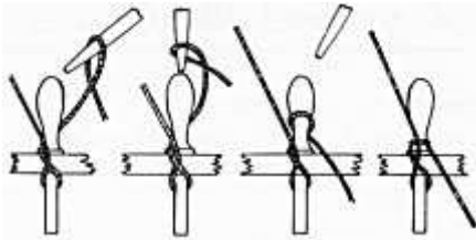
Fig.66 Belegen eines Tanes an einem Belegnagel
